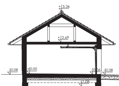
Przekrój
